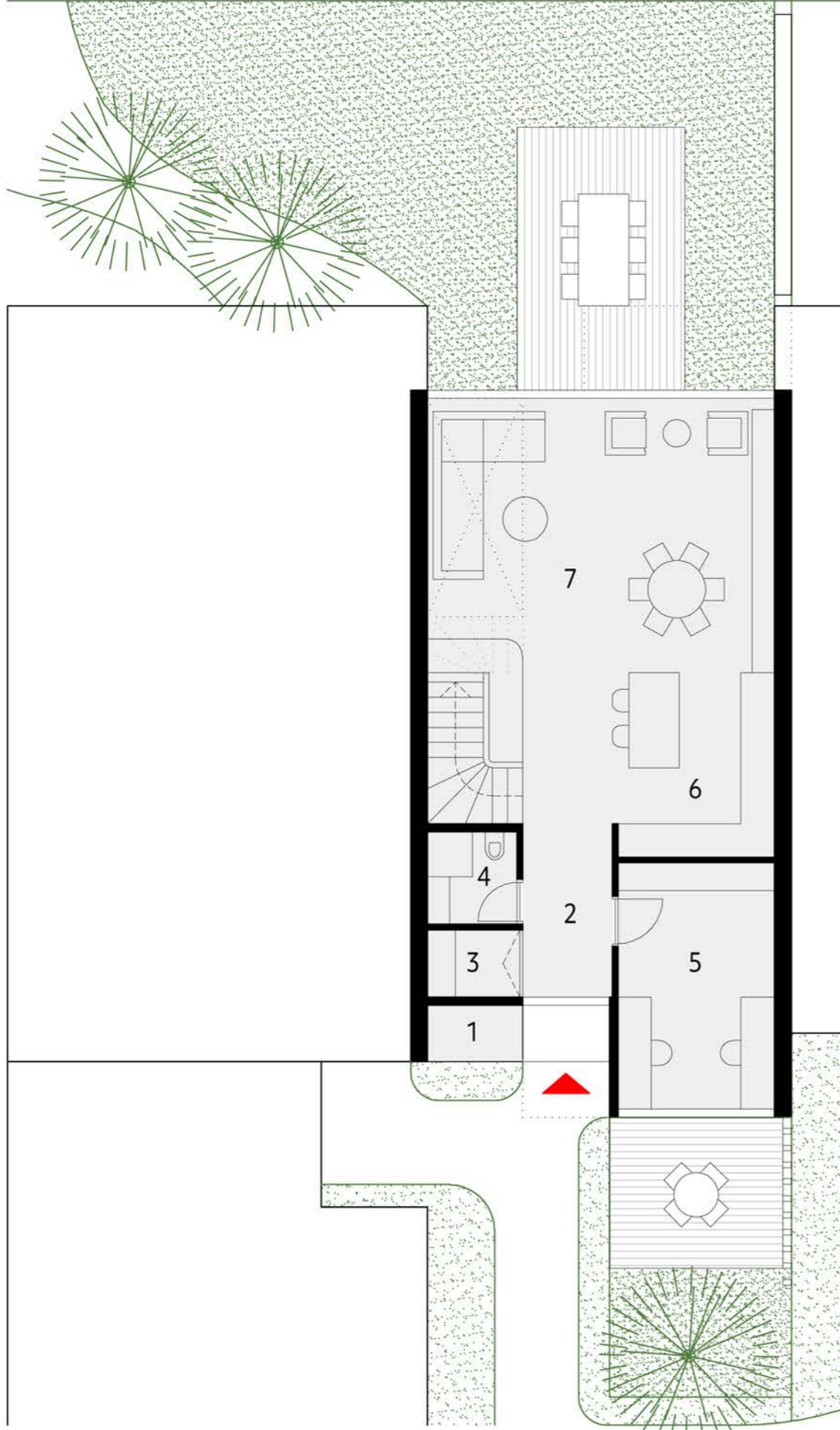
Zemin Kat Planı 1/100
