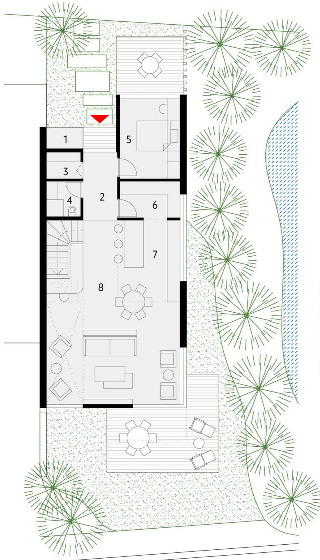
Zemin Kat Planı 1/100
